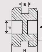
Vista laterale
